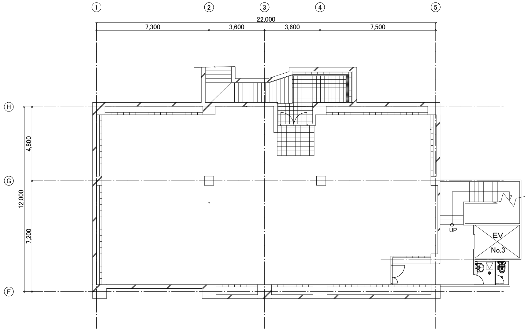
林英ビルB1F 平面図 1/150
